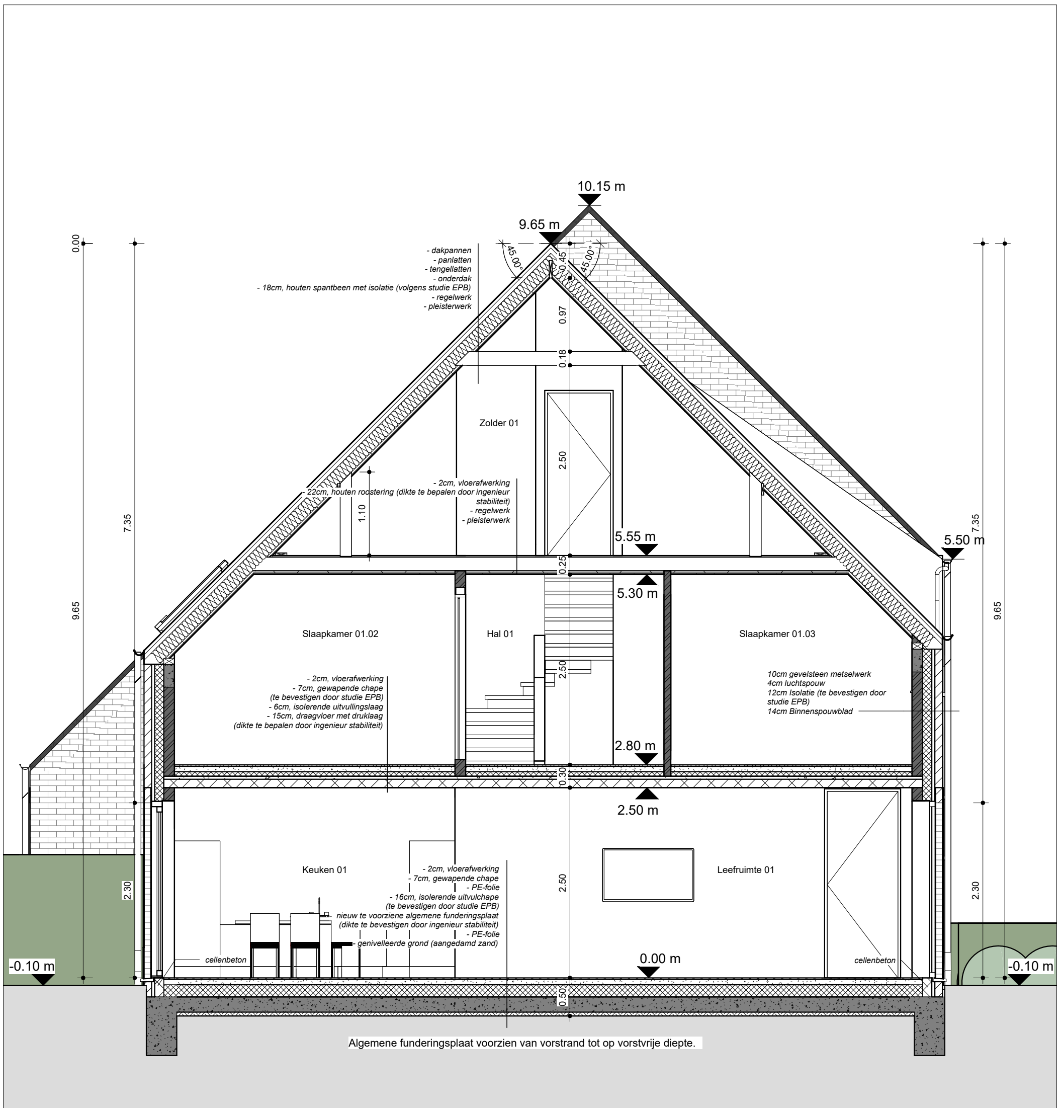
Snede D-D' - Lot 1
