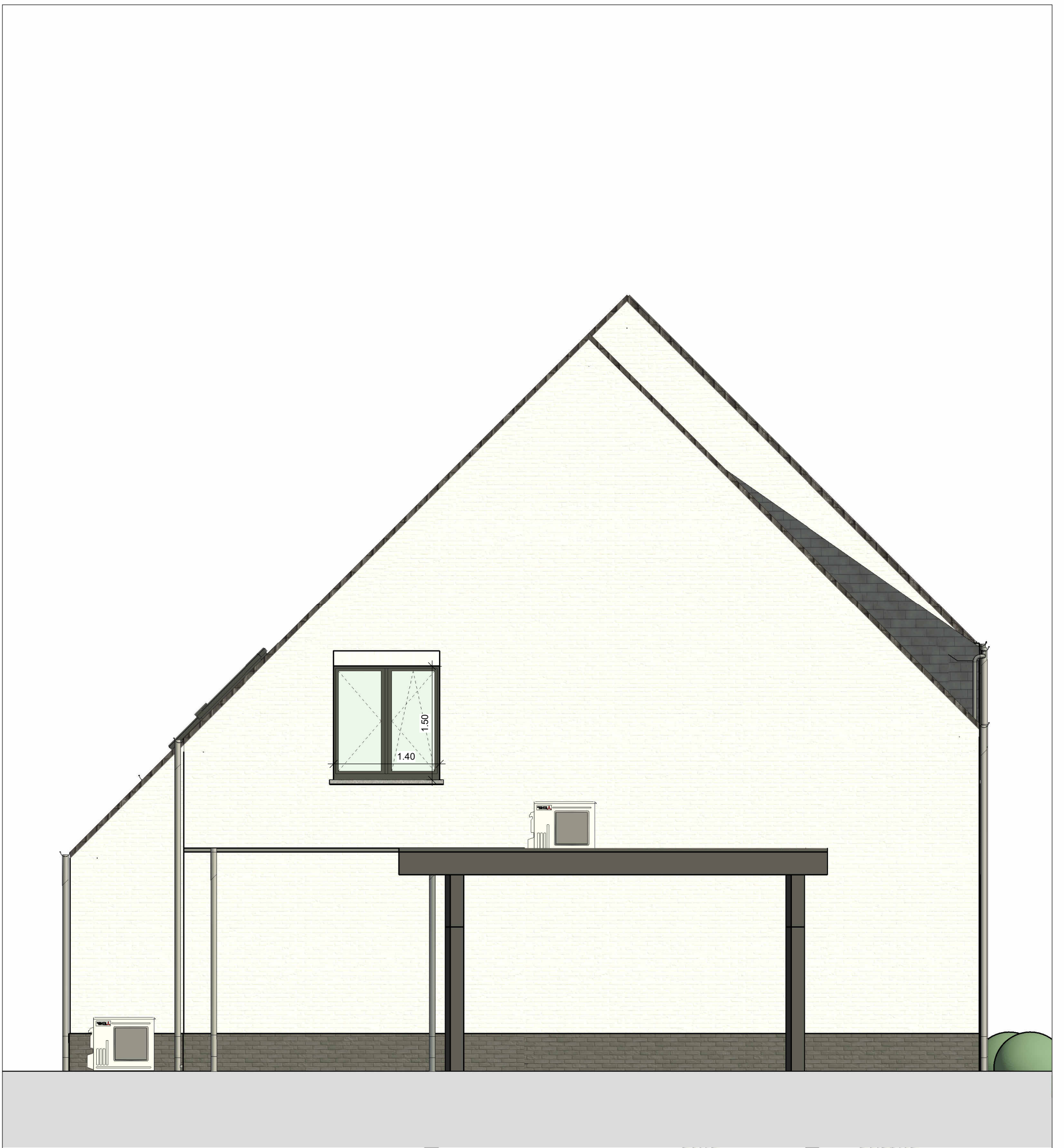
Linkerzijgevel - Lot 1
